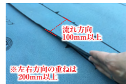
▲防水紙重ね巾の確認
